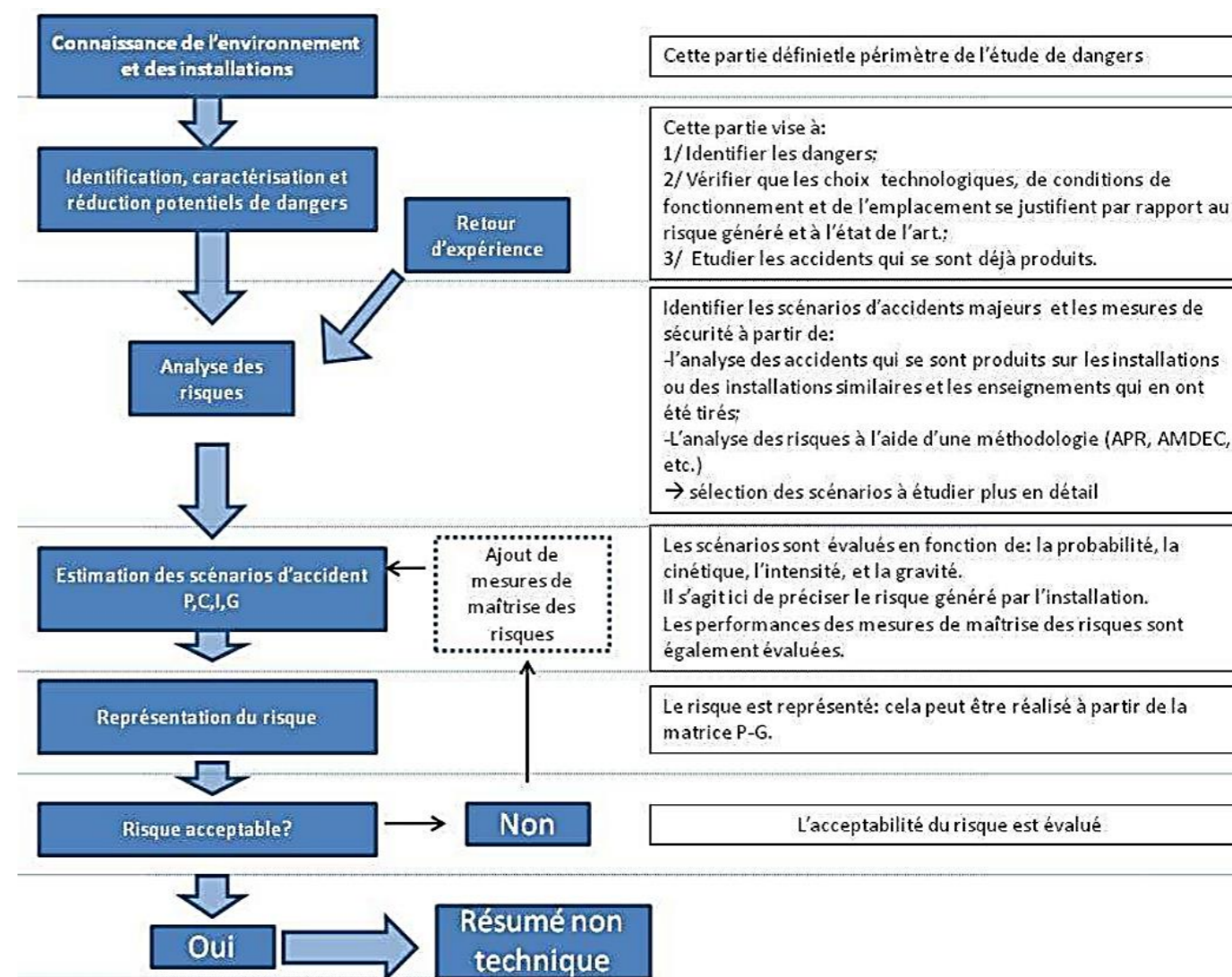
Figure 2 : Etapes et objectifs d'une étude de danger (Source : Guide technique sur l'élaboration de l'étude de dangers dans le cadre des parcs éoliens - INERIS)
