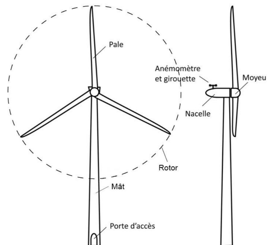
Figure 3 : Schéma simplifié d'un aérogénérateur
