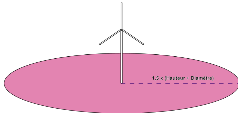
Figure 11 : Zone d'effet du phénomène de projection de glace
