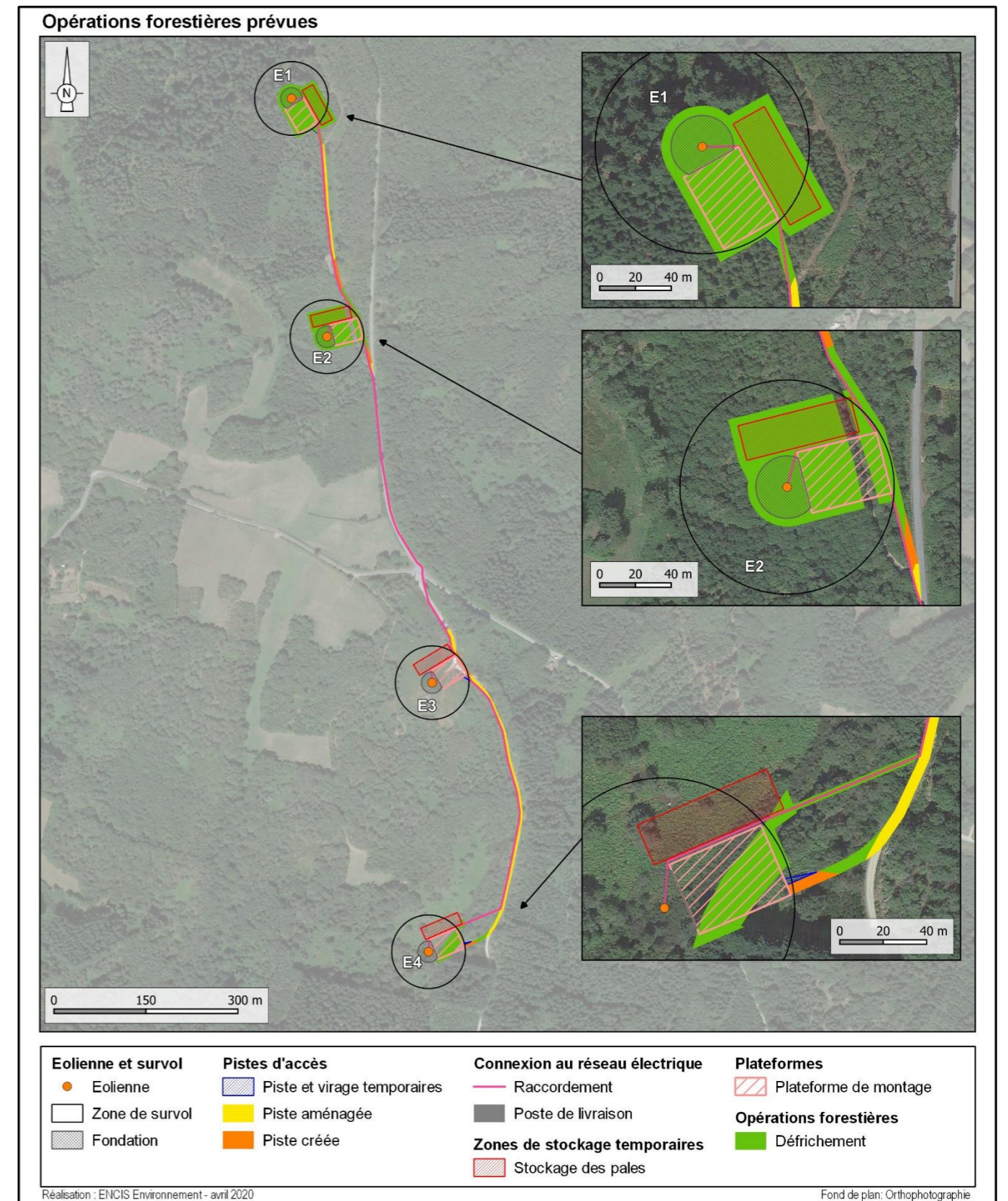
Plan du défrichage lors de la préparation du site
