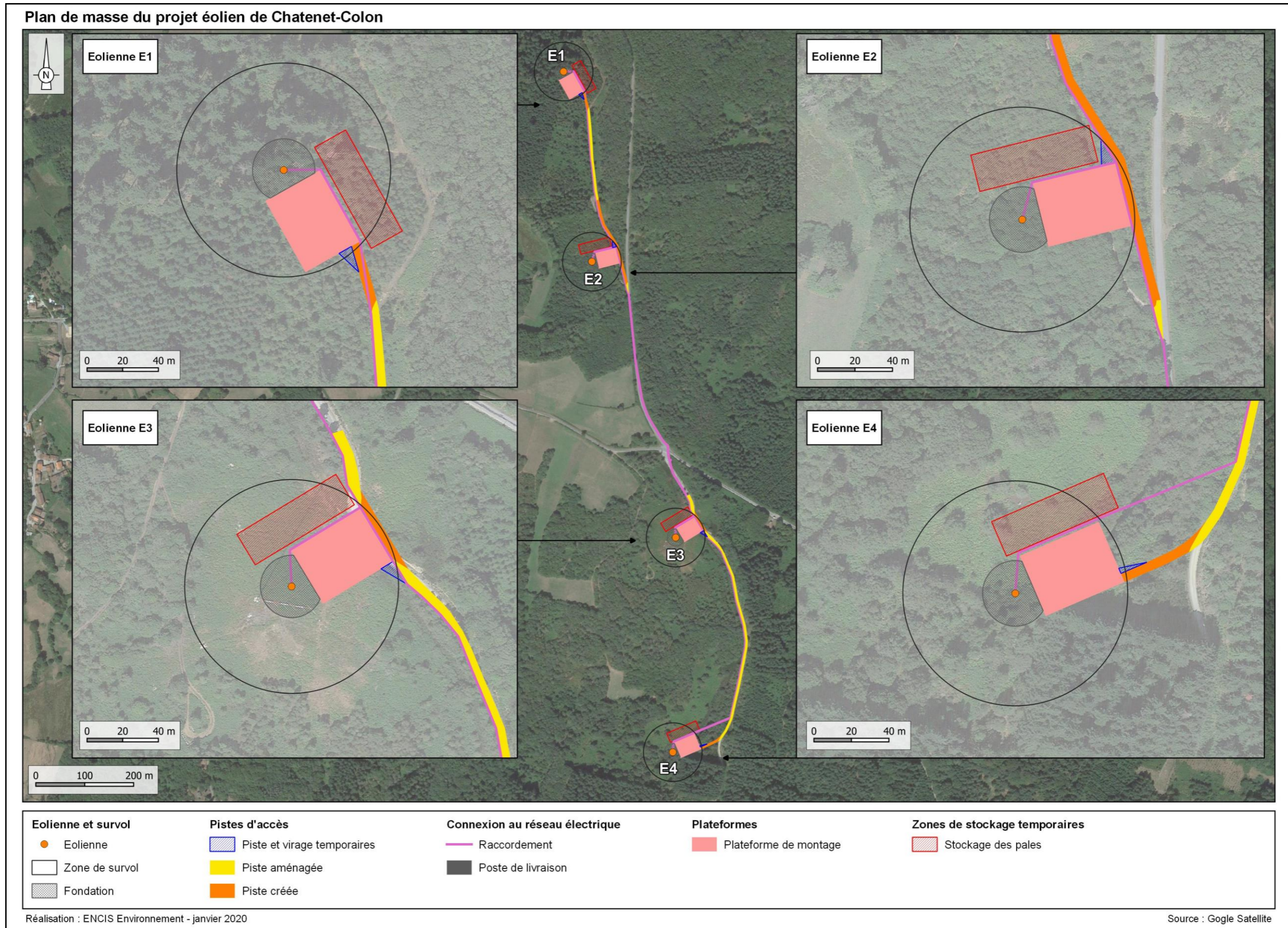
Plan de masse du projet éolien de Chatenet-Colon
