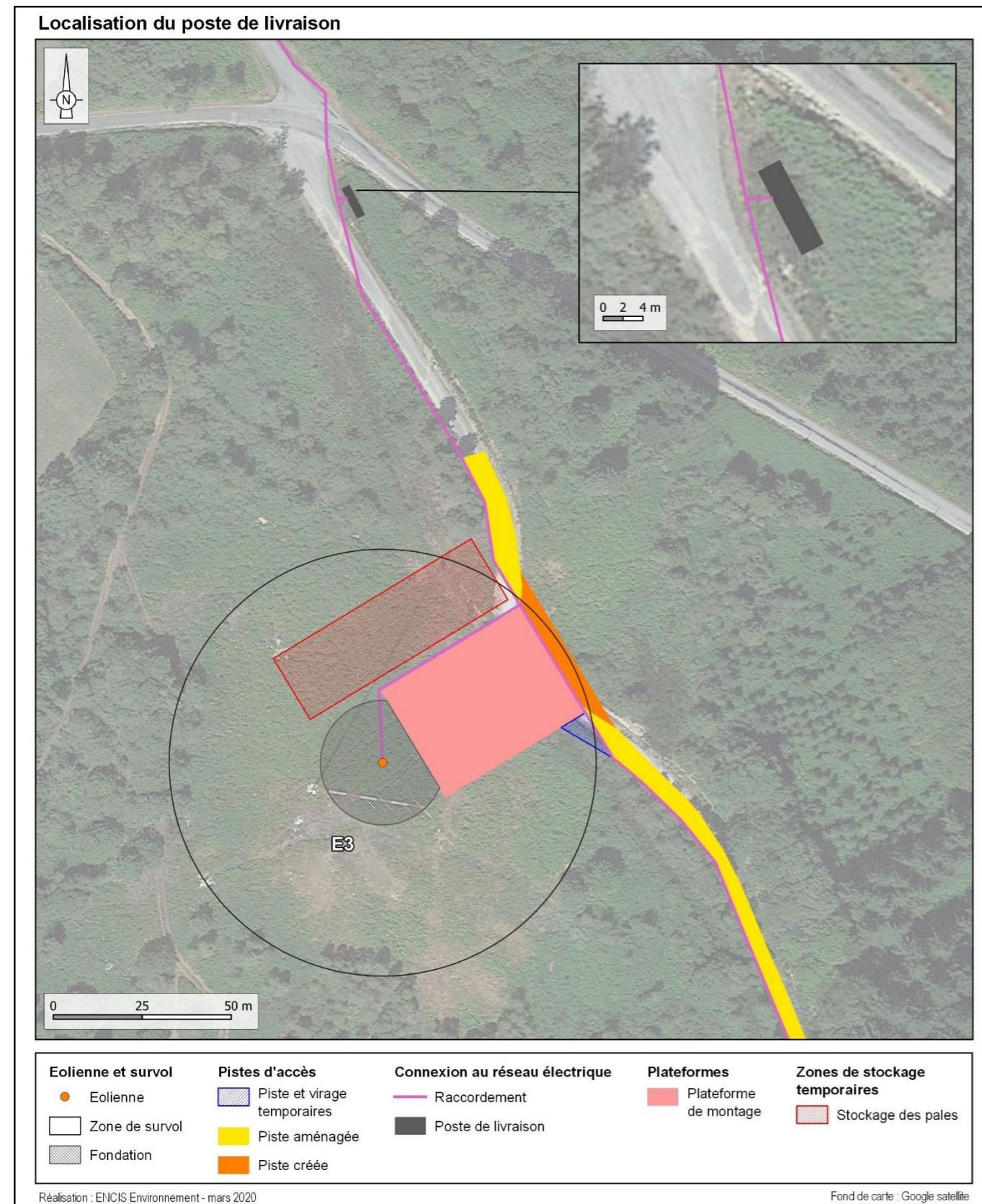
Localisation du poste de livraison
